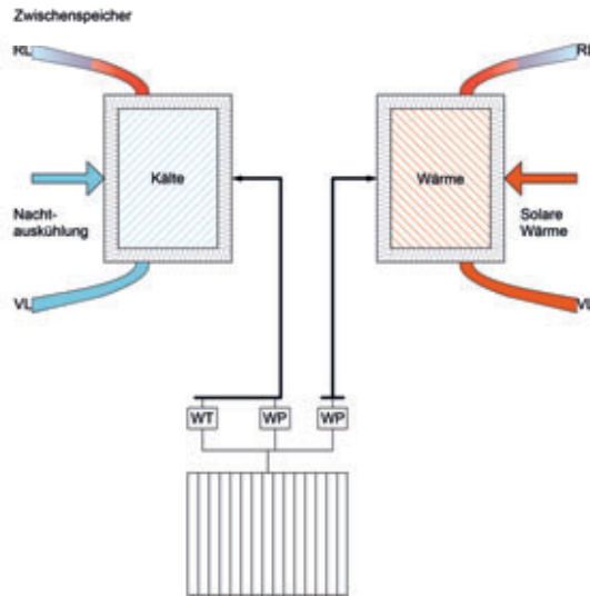
Einfache kostenarme Energieversorgung über Erdwärme
