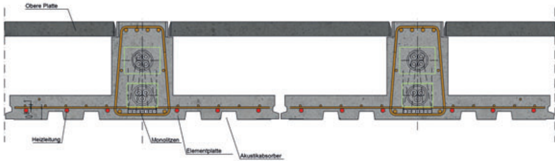
Sandwichquerschnitt mit getrennten Bauteilmassen und oberflächennahen Rohrleitungen
