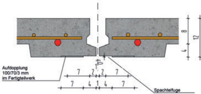
Detail für die Ausbildung der Fuge bei gestrichener Oberfläche
