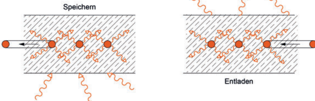
In Verbindung mit eingelegten Rohrregistern wird der Betonquerschnitt zu einem aktiven Speicher
